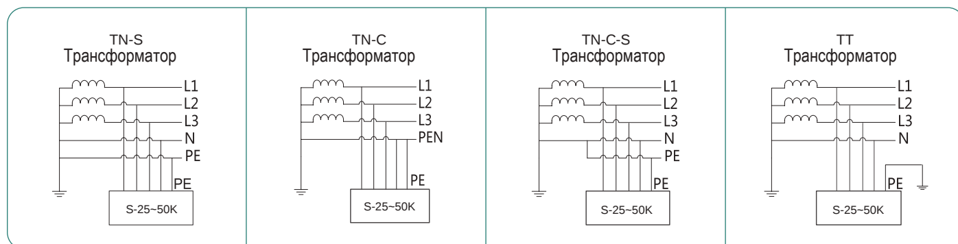
Малюнок 3-2 Застосовні типи мережі
