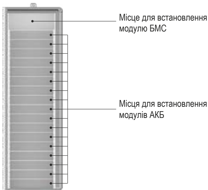
Шафа (вигляд спереду)
